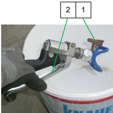
Abb. 58: Düsengriff
