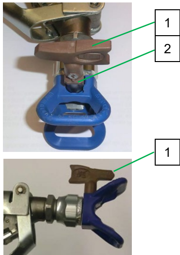
Abb. 27: Düse einsetzen
