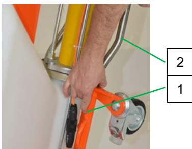
Abb. 69: Griff entfernen
