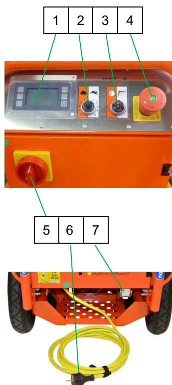
Abb. 7: Baugruppe Schaltschrank
