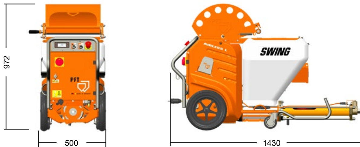
Abb. 2: Maßblatt
