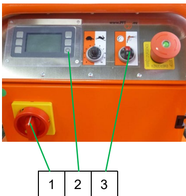
Abb. 52: Wiederaufschaltung
