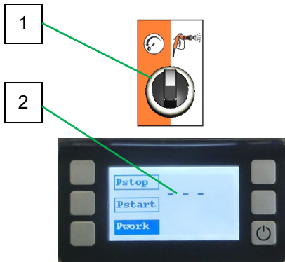
Abb. 57: Drehrichtung ändern
