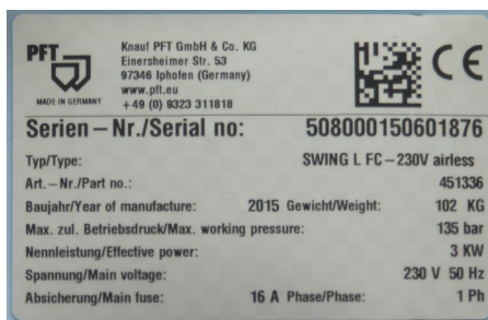
Abb. 3: Typenschild
