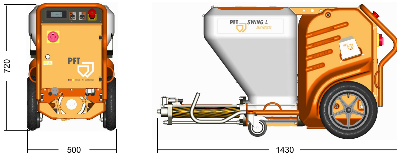
Abb. 1: Maßblatt
