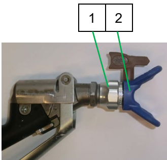
Abb. 63: Spritzdüse
