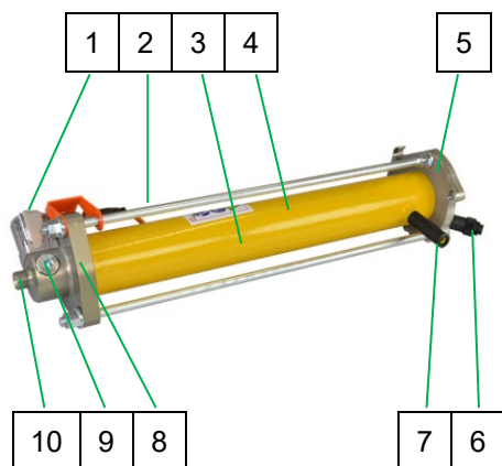
Abb. 6: Baugruppe Pumpeneinheit
